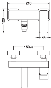
消光黑 方形浴用龍頭 8.24.022MB $7,800
