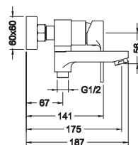
消光黑 方形浴用龍頭 8.24.022MB $7,800
