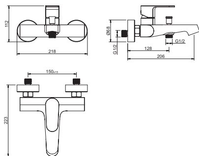
鉻色 浴用龍頭 8.04.022CH $7,600
