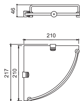
消光黑 轉角玻璃架 (帶護欄) 7.03.074MB 210*210*h46 mm $1,300
