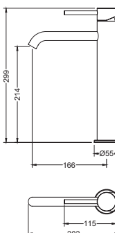
消光黑 加高面盆龍頭 8.09.112MB $7,400
