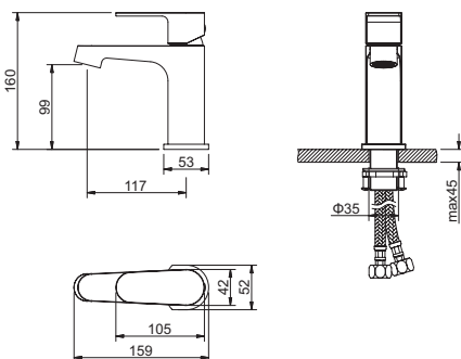
槍灰色 面盆龍頭 8.04.011BGM $5,800
