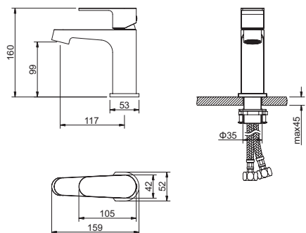
鉻色 面盆龍頭 8.04.011CH $4,900
