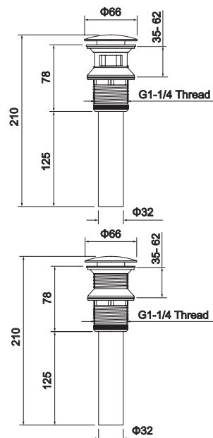
金色 歐規按壓落水頭 (有溢水孔) 6.PU.001PG $1,200
