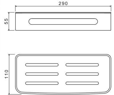
單層方型籃 ABS+ 不鏽鋼 (附掛勾) 0.10.027ST 290*110*h55 mm $1,050
