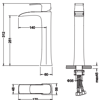
加高面盆龍頭 8.62.02 $8,400
