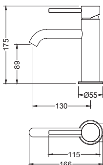
消光黑 面盆龍頭 8.09.011MB $5,900
