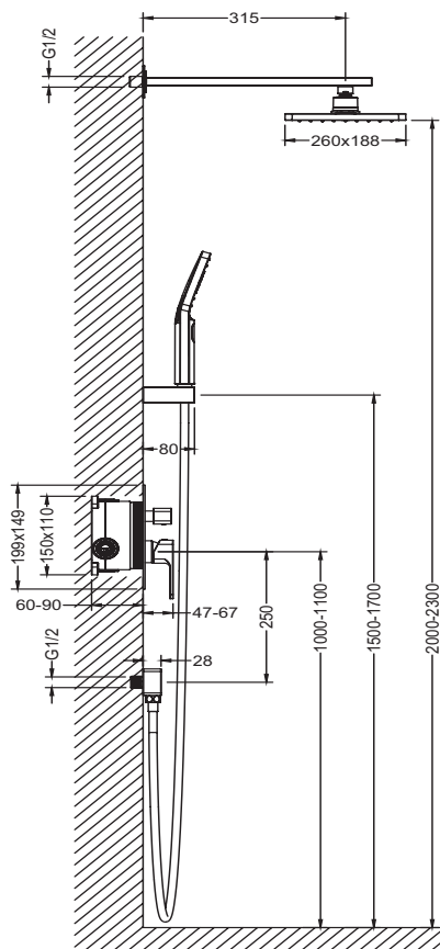
消光黑 埋壁式浴用龍頭 8.24.2201MB $13,600
