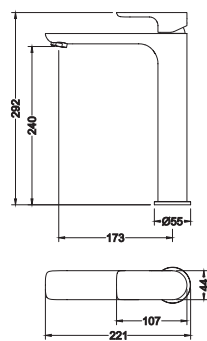
加高面盆龍頭 8.25.012 $8,000
