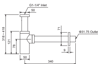
歐式 TP 管組 X-6.TP 管 $2,000
