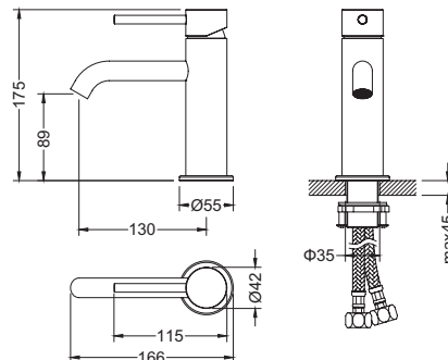
玫瑰金 面盆龍頭 8.09.011PRG $7,100
