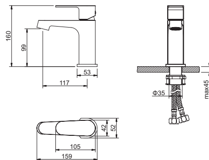
拉絲金 面盆龍頭 8.04.011BG $5,800
