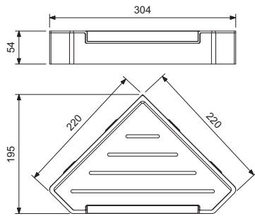
單層轉角籃 ABS+ 不鏽鋼 (附刮刀) 0.10.039ST 220*220*h54 mm $1,300
