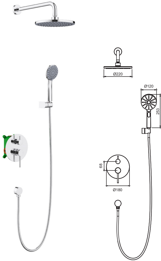
埋壁式浴用龍頭 8.09.2201 $8,000
