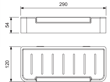
單層方型籃 ABS+ 不鏽鋼 (附刮刀) 0.10.040ST 290*120*h54 mm $1,300
