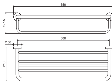
不鏽鋼雙層置物架 7.04.058ST 650*210*h127.5 mm $2,200
