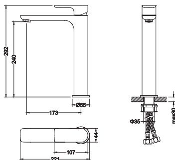
金色 加高面盆龍頭 8.25.012PG $8,800
